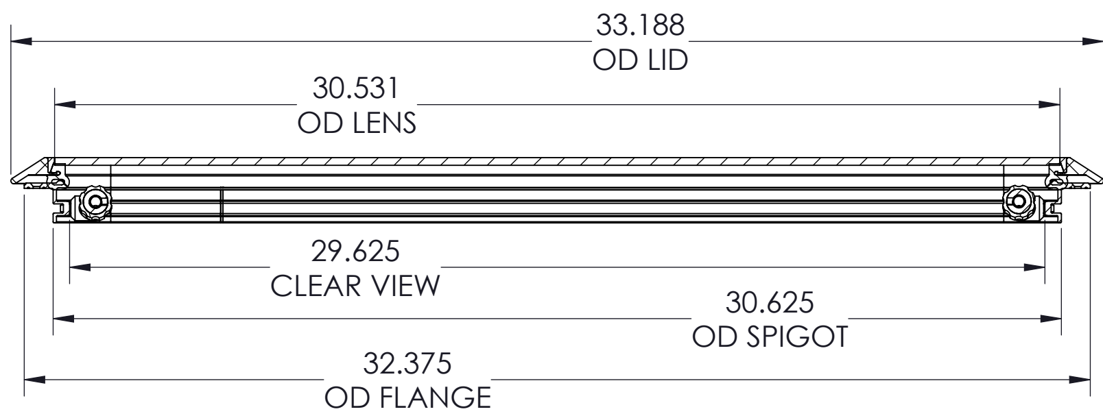
SECTION A-A
